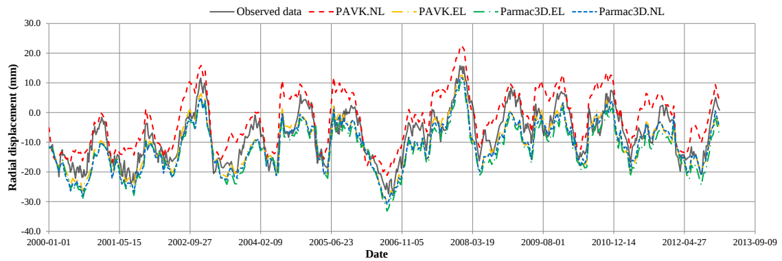
a) Pendulum CB2
